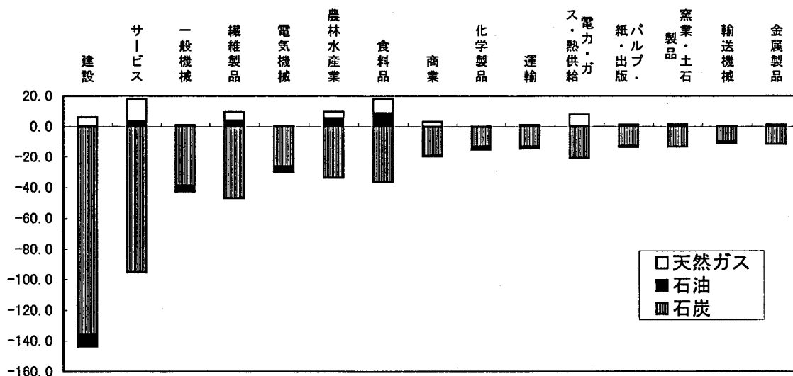
図3(b) 中国(1992年)で日本の1990年技術での二酸化炭素削減量 単位は炭素換算100万トン、総削減は450
