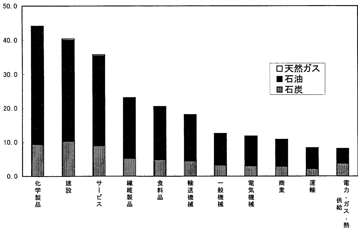
図1(a) 日本(1970年)での二酸化炭素炭素排出量 単位は炭素換算100万トン, 総排出量は244
