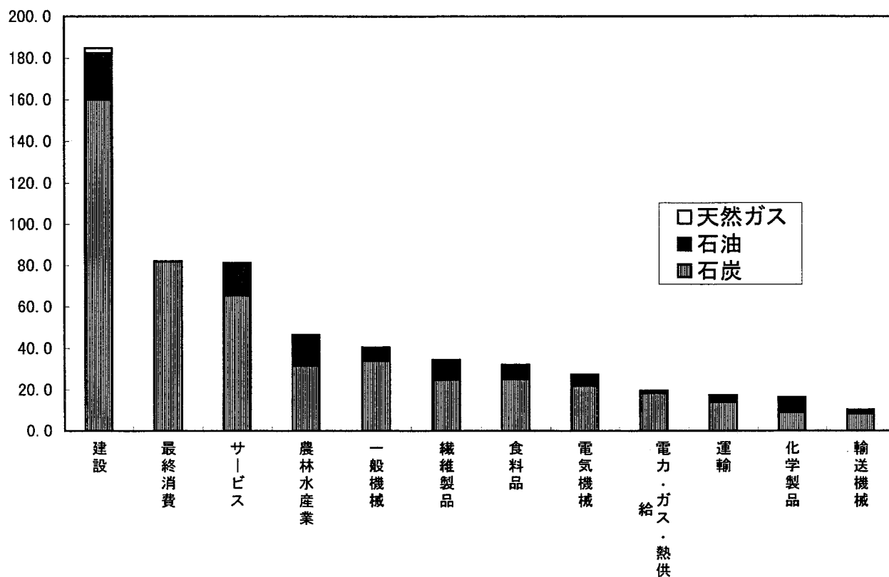
図2(a) 中国(1987年)での二酸化炭素発生量 単位は炭素換算100万トン, 総排出は604
