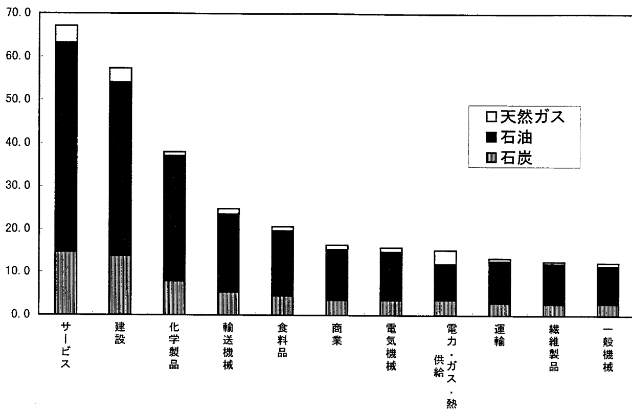
図 1(b) 日本(1980年)での二酸化炭素発生量 単位は炭素換算100万トン、総排出は291
