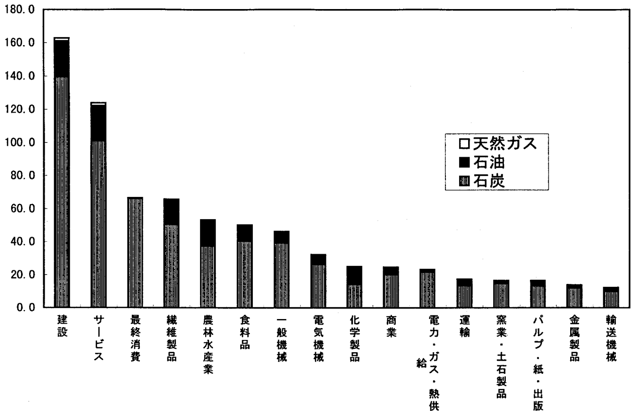
図 2(b) 中国(1992年)での二酸化炭素発生量 単位は炭素換算100万トン、総排出は734
