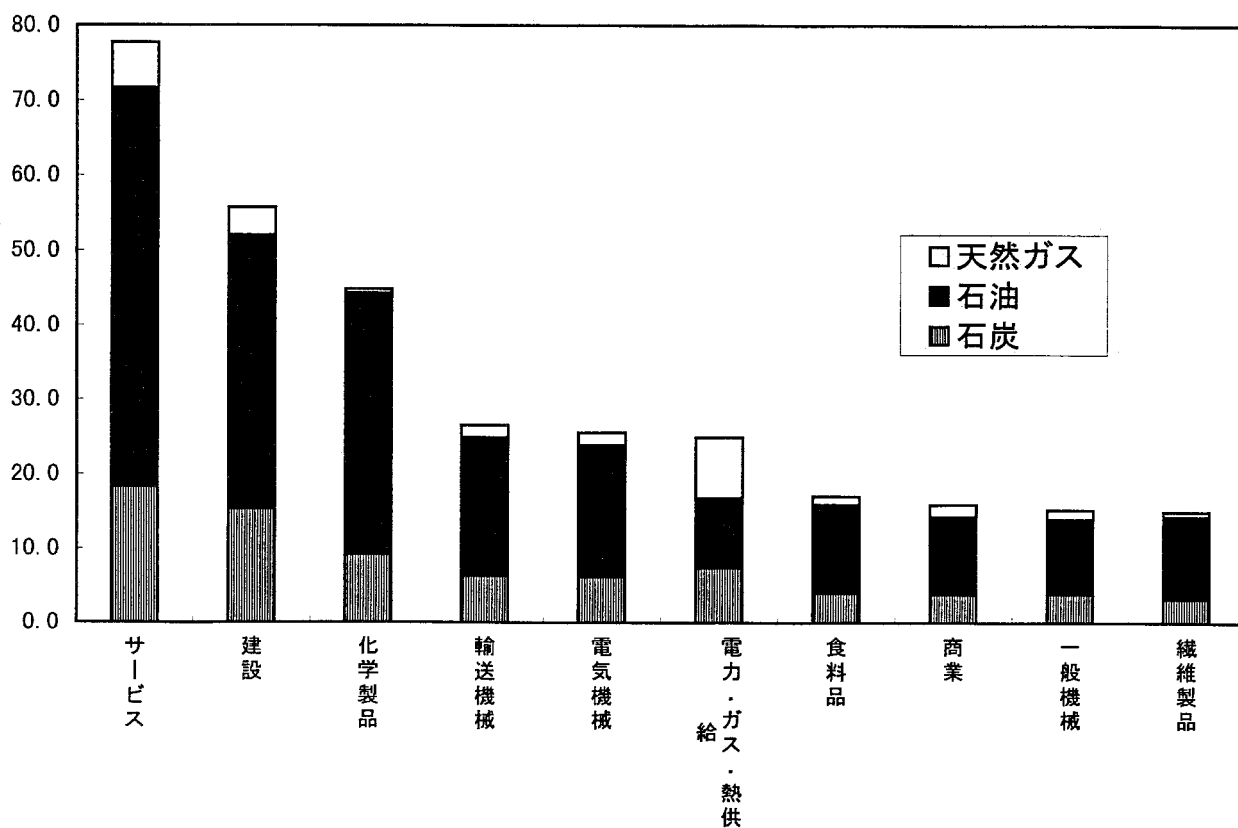
図 1(c) 日本(1990年)での二酸化炭素発生量 単位は炭素換算100万トン、総排出は333
